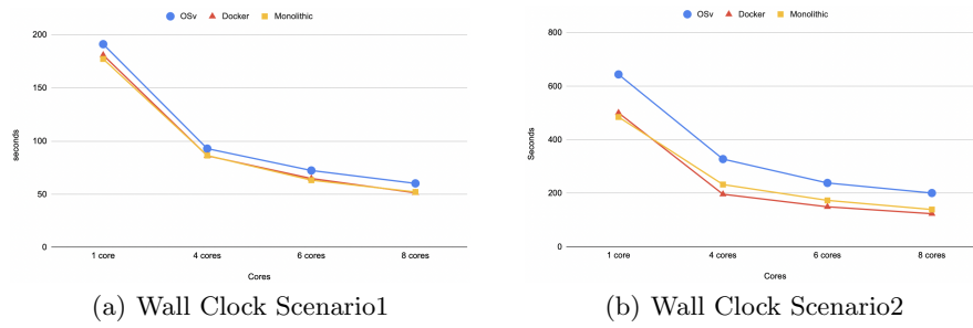
Fig. 2. Bootup times
