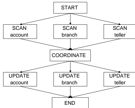
Fig. 4. Informix example
